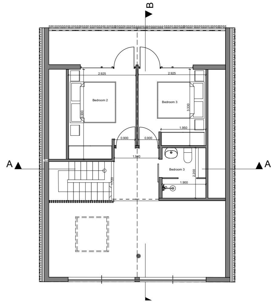
1. 2. Floor 1:100
