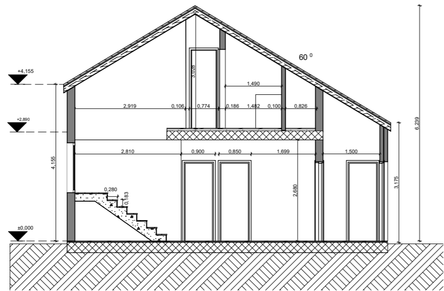
Section BB 1:100
