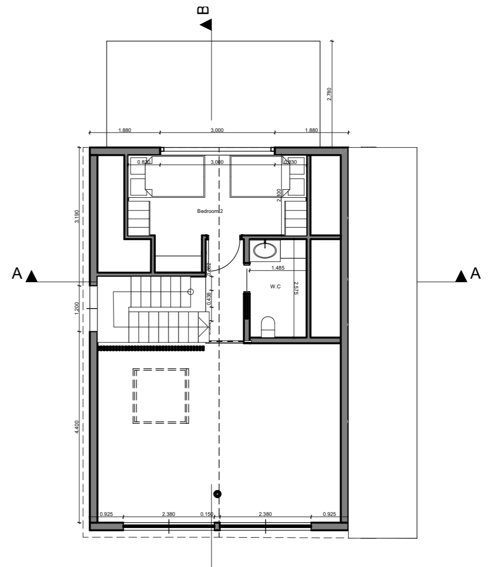
1. 2. Floor 1:100
